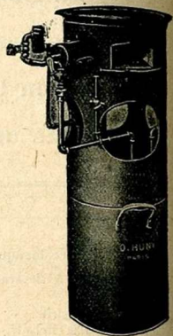
FOUR A RIVETS AUX HUILES LOURDES
